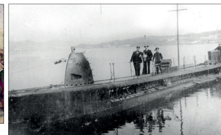
Субмарина «Касатка». 1904 г.
